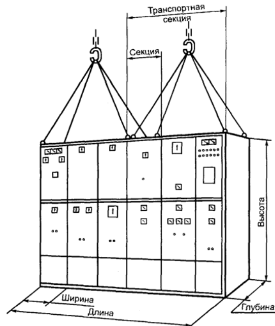
Рисунок С.4 — НСУ заводского изготовления многошкафного типа
