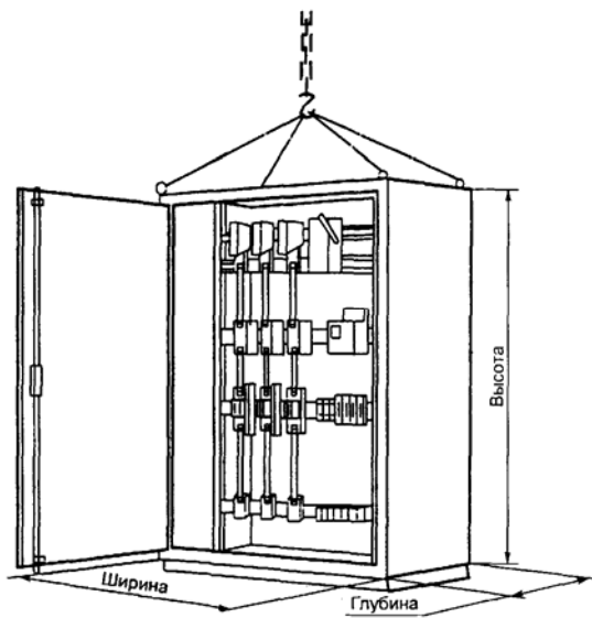
Рисунок С.1 — НСУ заводского изготовления открытого типа
