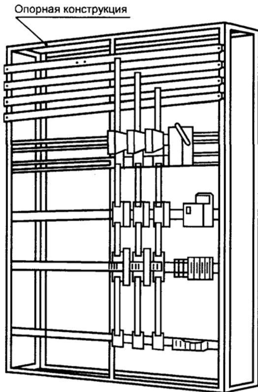
Рисунок С.1 — НСУ заводского изготовления открытого типа
